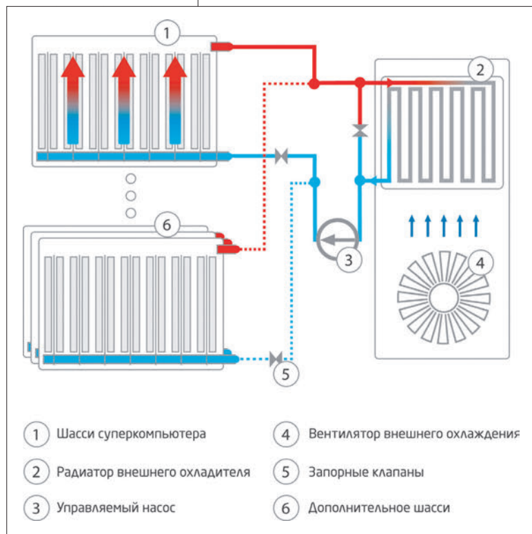
Рис. 1. Схема погружного охлаждения
